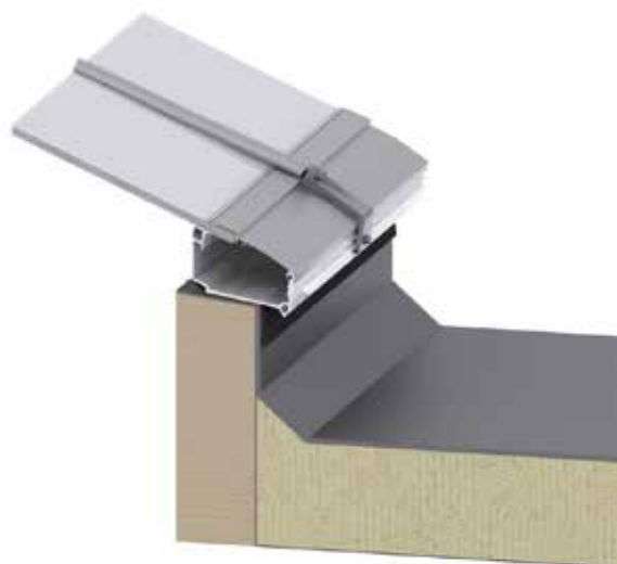
Montage op verlijmd houtproducten
